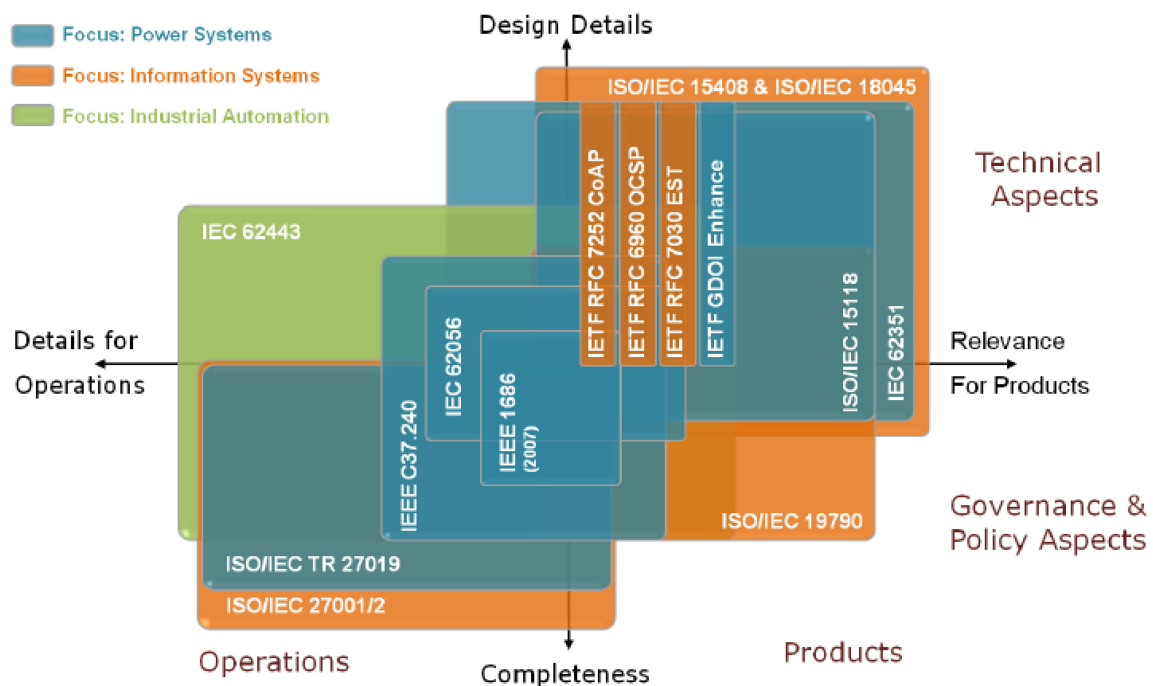
Abbildung 5: Smart Grid Normenlandschaft und deren Kategorisierung
