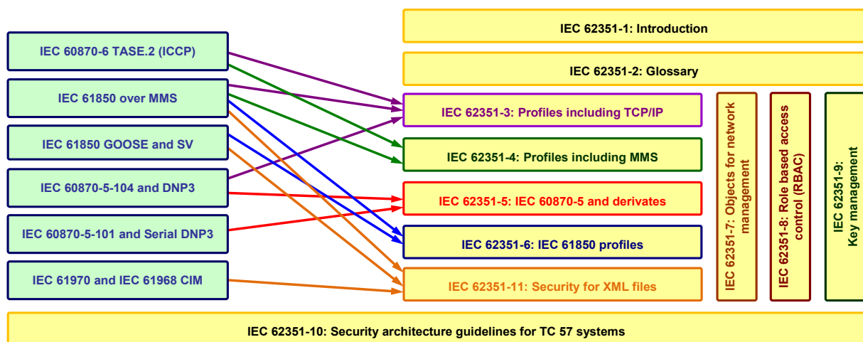
Abbildung 7: IEC TC 57 Kommunikationsstandards und ihre Relation zu den Teilen der IEC 62351 [Quelle: IEC]
