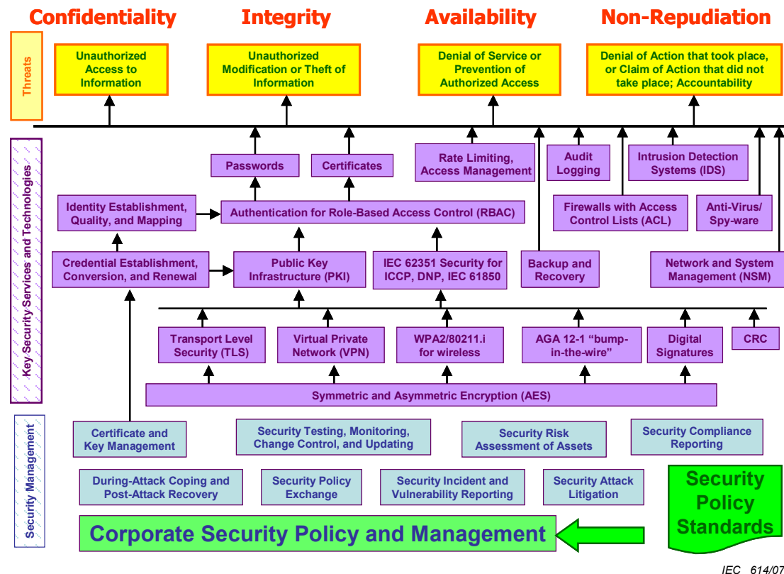
Abbildung 8: Sicherheitsanforderungen, Bedrohungen, Gegenmaßnahmen und Management [Quelle: IEC 62351-1]
