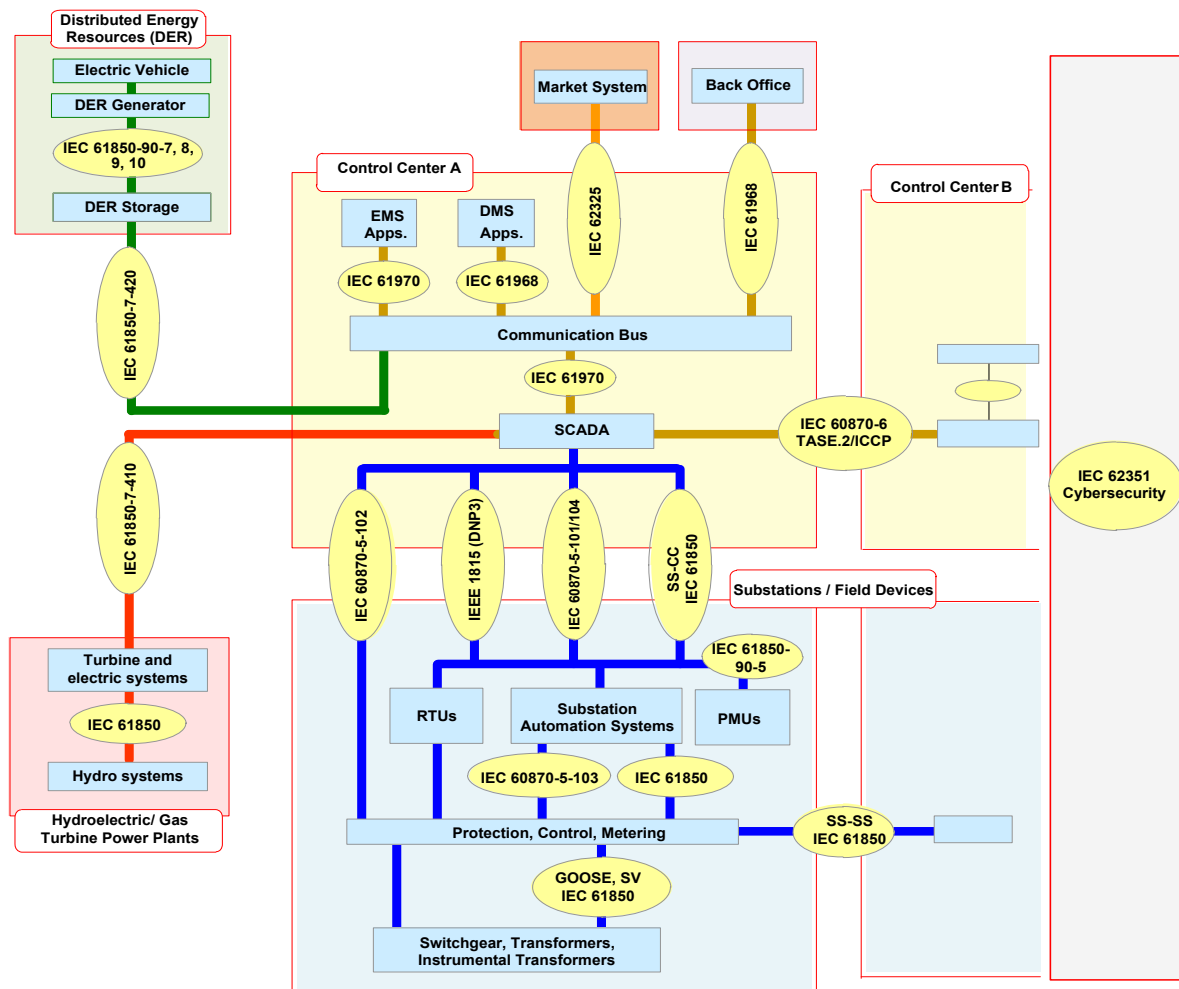
Abbildung 6: IEC TC 57 Architektur von Kommunikationsstandards [Quelle: IEC 62351-10]
